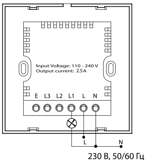
Схема электрических соединений (CPC-1 и CPC-2.5)
