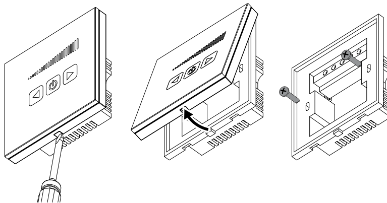
Монтаж сенсорного регулятора скоростей
