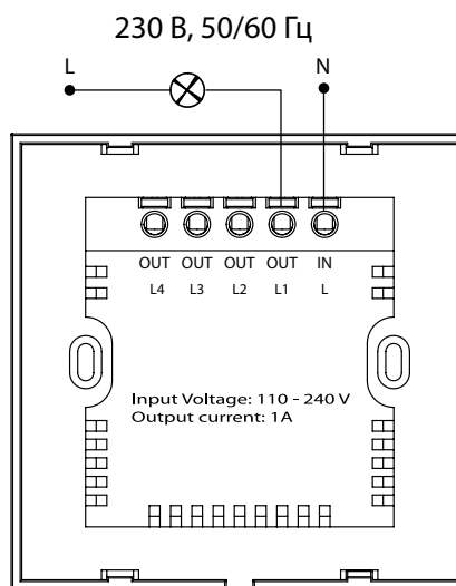
Схема электрических соединений (только для CPC-1)
